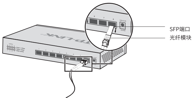
图3-2 SFP端口连接示意图
