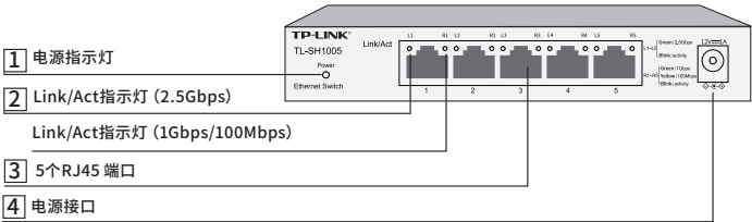
图1-1 TL-SH1005前面板示意图
