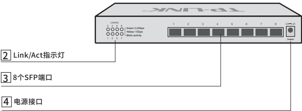
图1-6 TL-SH1008F后面板示意图
