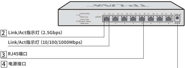
图1-4 TL-SH1008后面板示意图
